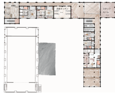
二階平面図 1/1500
