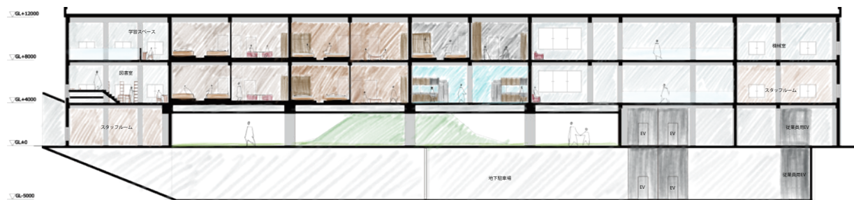
東西断面 1/500
